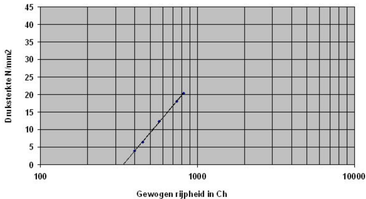
IJkgrafiek koude gietbouw
